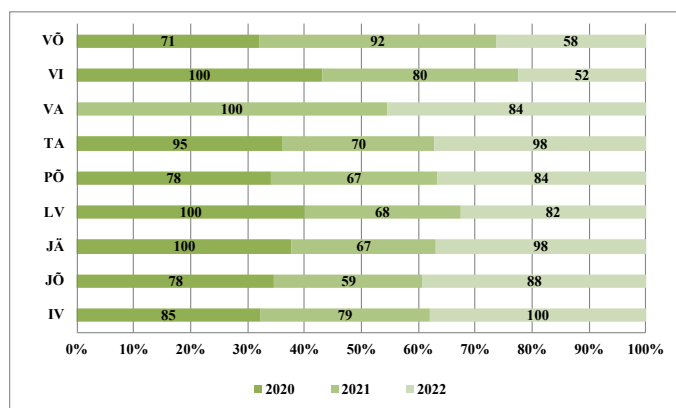
Joonis 12. Mutatsiooni G143A sagedused (%) märklaudvalgus CytB Z. tritici populatsioonis 2020 - 2022 a
