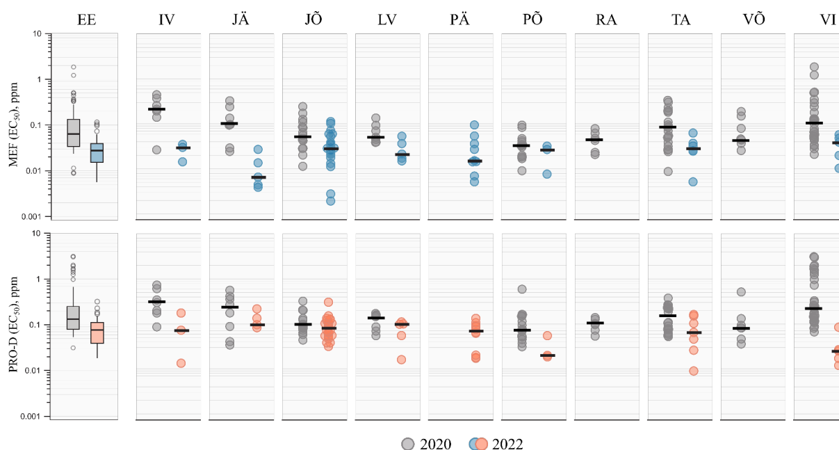
Joonis 5. Rcc mefentriflukonasooli (MEF) ja protiokonasool-destio (PRO-D) EC_{50} (ppm) taseme varieeruvus maakondade lõikes. ●, ●, ● tähistab isolaati; – karpdiagrammil ja hajuvusdiagrammil olev joon tähistab mediaankeskmist EC_{50} väärtust. Maakondade lühendid nagu joonis 1.
