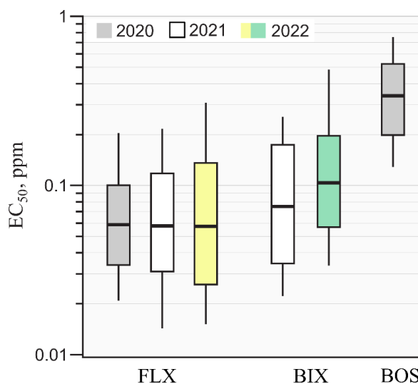
Joonis 10. Fluksapüroksoadi (FLX), biksafeeni (BIX) ja boskaliidi (BOS) EC_{50} kontsentratsioonid (ppm) aastatel 2020-2022 Zt Eesti populatsioonis. Karpdiagrammil olev joon tähistab EC_{50} mediaankeskmist väärtust.
