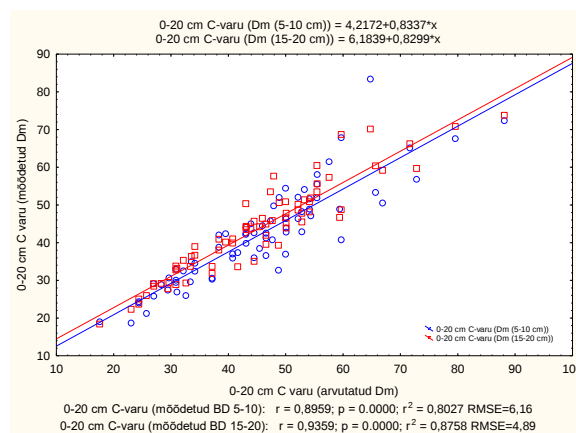
Joonis 3. Seos mõõdetud ja arvutatud lasuvustiheduse kaudu arvutatud 0-20 cm mullakihi C varude ( t \cdot ha^{-1} ) vahel
