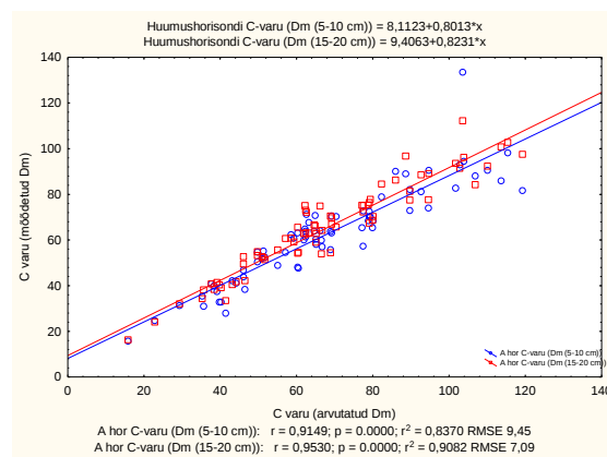
Joonis 2. Seos mõõdetud ja arvutatud lasuvustiheduse (Dm) kaudu arvutatud huumushorisondi (A hor) C varude ( t \cdot ha^{-1} ) vahel
